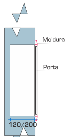
Detalhe da parede para conjunto embutido
